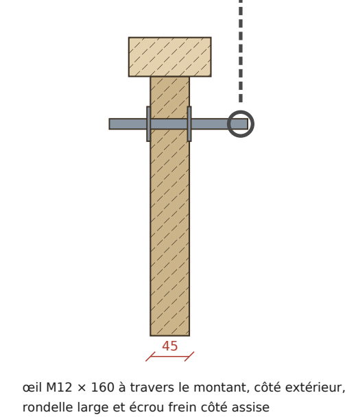
D6 — ATTACHE SUR LE BANC 1:6
