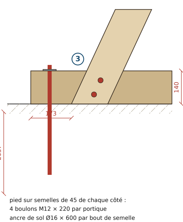
D7 — TRACÉ DU PIED 1:32
