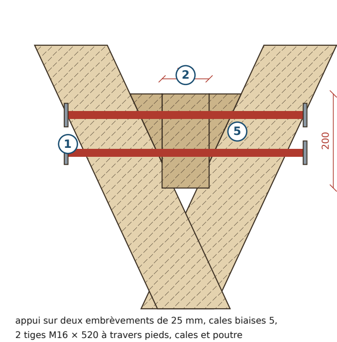
D1 — TÊTE D'A 1:8
