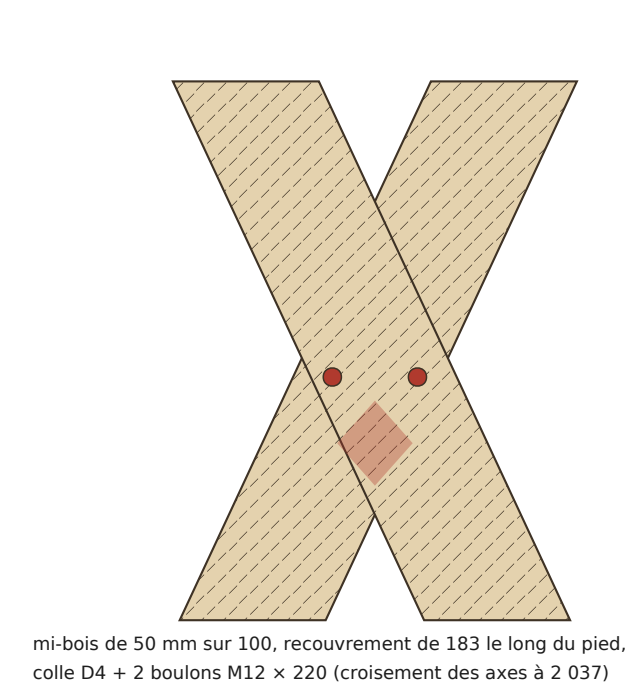
D2 — CROISEMENT DES PIEDS 1:8
