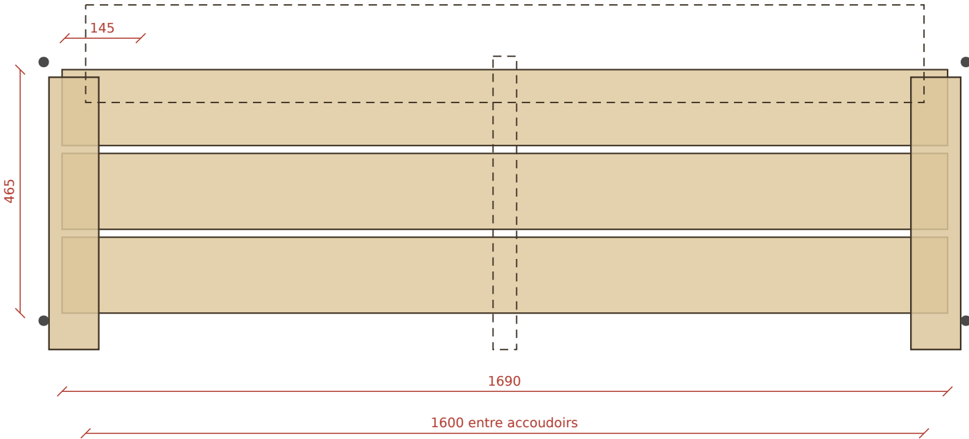
DESSUS DU BANC 1:10
