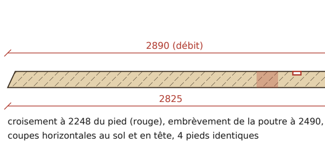
D7 — TRACÉ DU PIED 1:32
