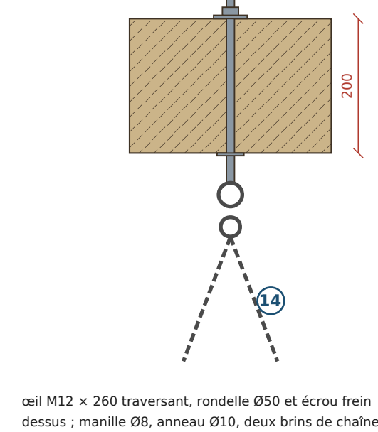
D5 — ŒIL DE POUTRE 1:8
