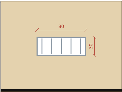
D6 — AÉRATION 1:3
