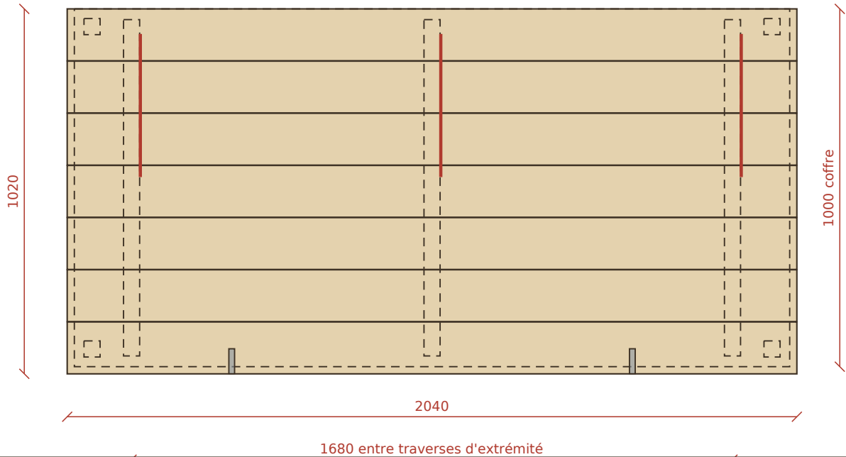
DESSUS, COUVERCLE FERMÉ 1:15
