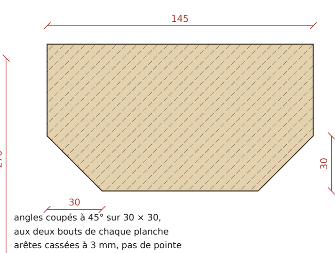
D4 — COIN DE PLANCHE 1:2
