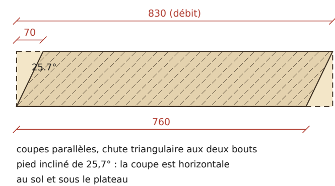
D2 — TRACÉ DU PIED 1:10
