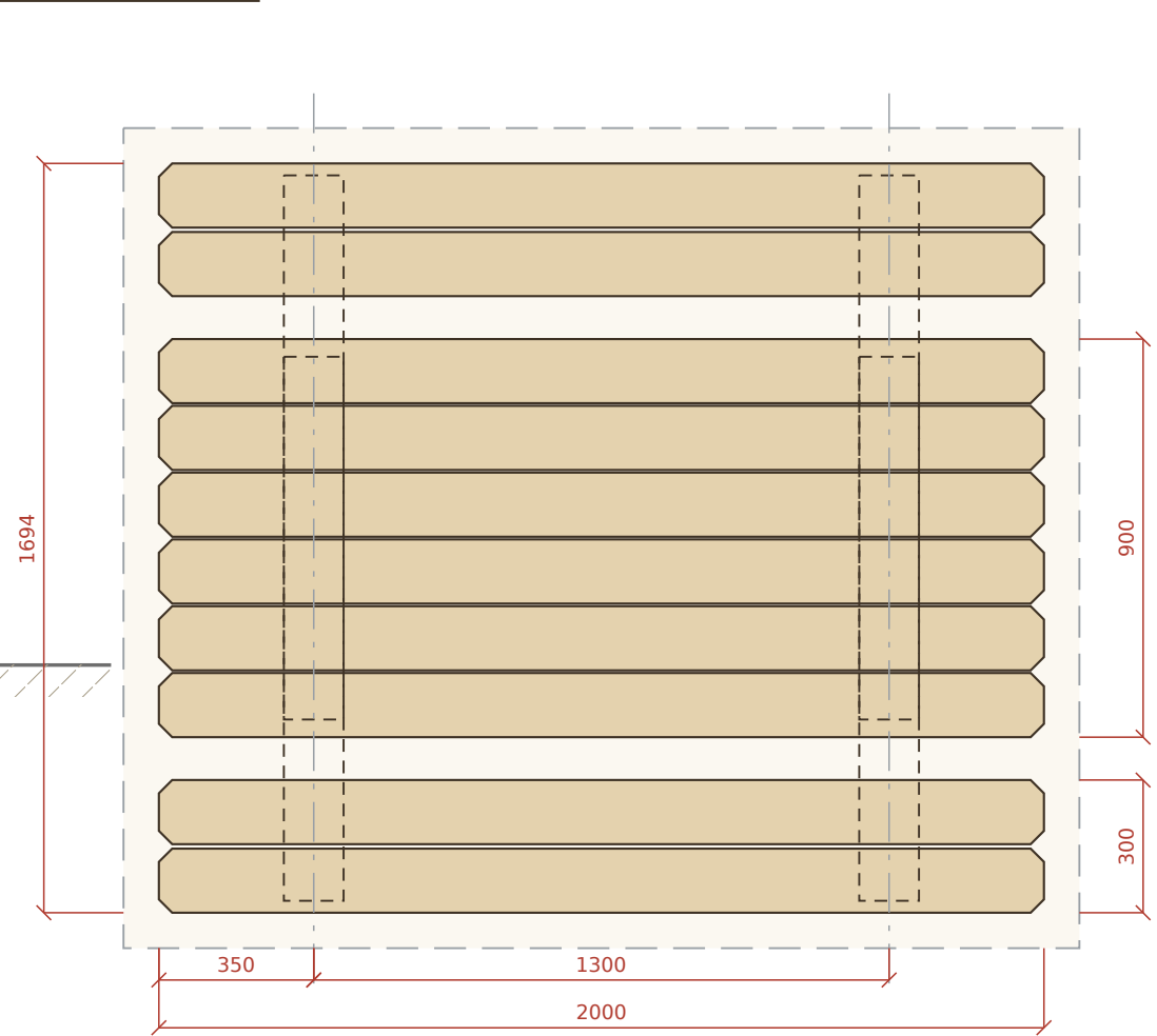
VUE DE DESSUS 1:18
