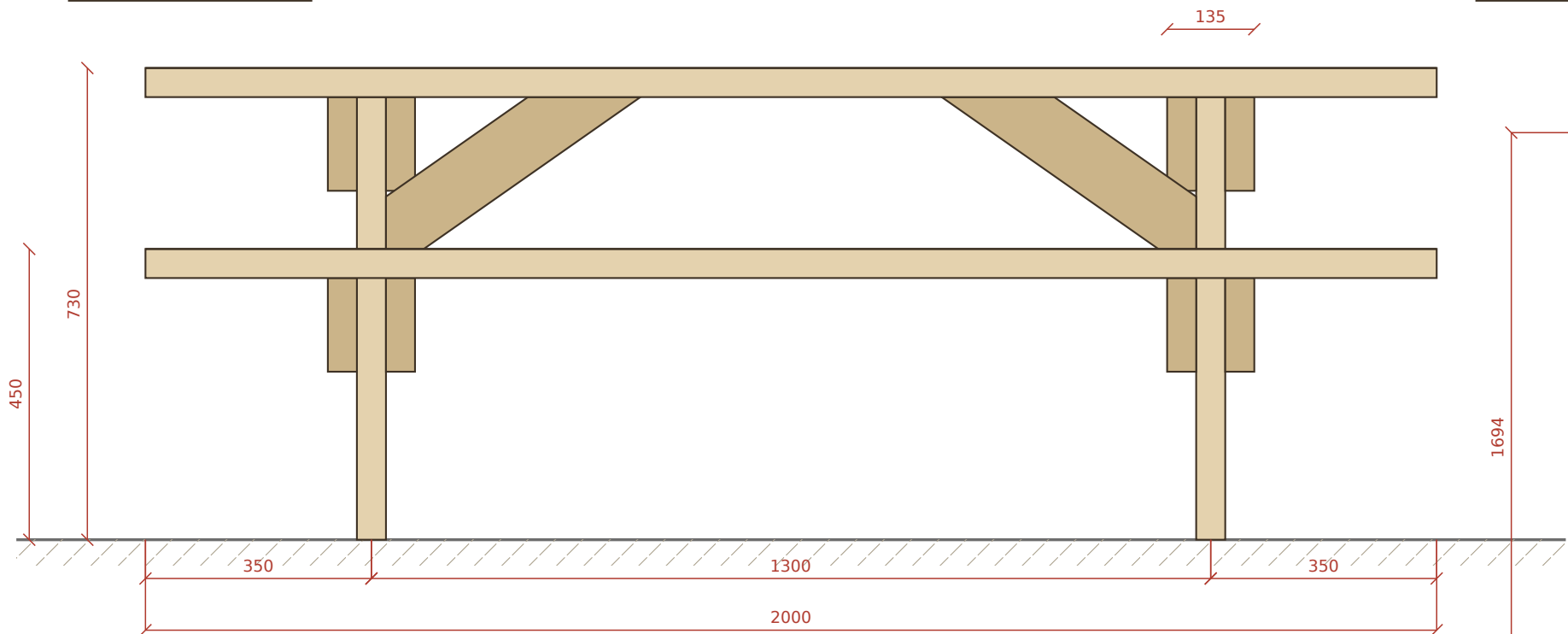
VUE DE BOUT 1:10
