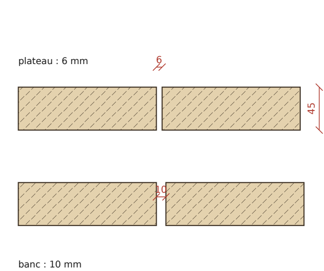
D5 — JEUX ENTRE PLANCHES 1:4
