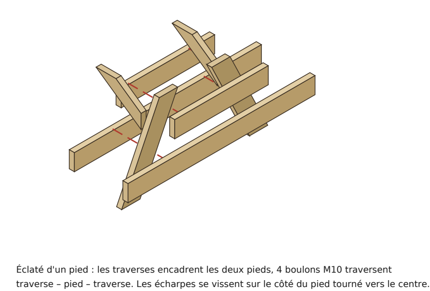
D6 — ÉCLATÉ D'UN PIED EN A
