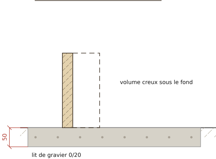
D3 — PIED DE CAISSE éch. 1:6
